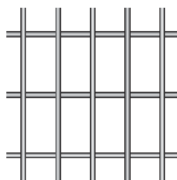
Art. 9 Filo ø: 2,85 Maglia: 50 x 30 Pannello: 1200 x 2400
