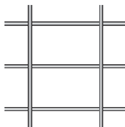
Art. 10 Filo ø: 2,85 Maglia: 50 x 100 Pannello: 1200 x 2400
