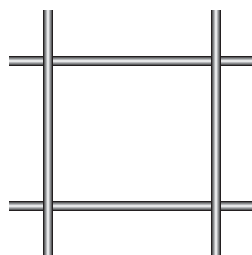
Art. 11 Filo ø: 4 Maglia: 100 x 100 Pannello: 1200 x 2400
