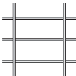
Art. 14 Filo ø: 4 Maglia: 50 x 100 Pannello: 1000 x 2400
