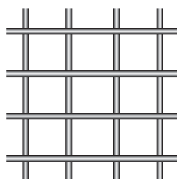
Art. 18 Filo ø: 4 Maglia: 40 x 40 Pannello: 1100 x 2200
