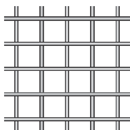
Art. 7 Filo ø: 2,85 Maglia: 30 x 30 Pannello: 1200 x 2400
